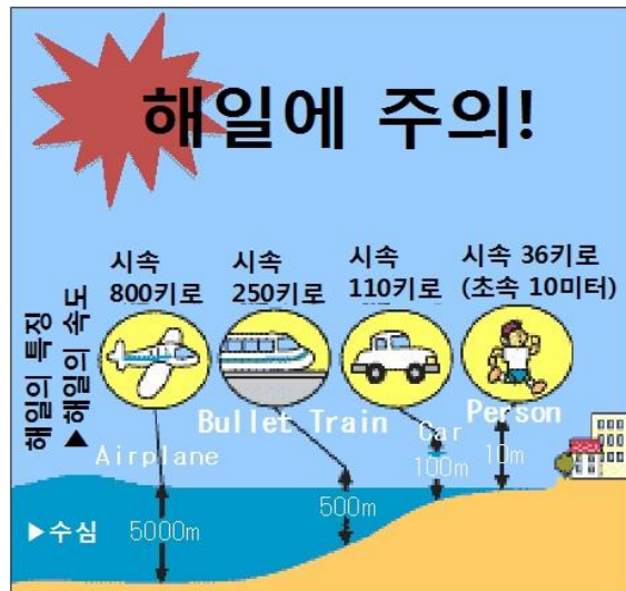
지진해일의 전파속도와 바다 깊이와의 관계
