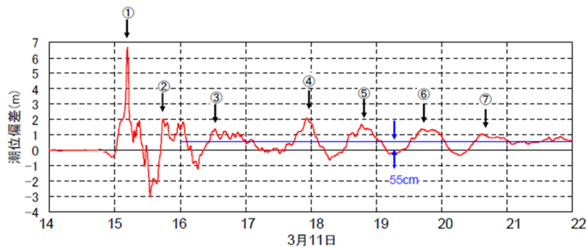
도-1 이와테 남부 앞바다 GPS 파도측량계로 파악된 해일의 초기파형
